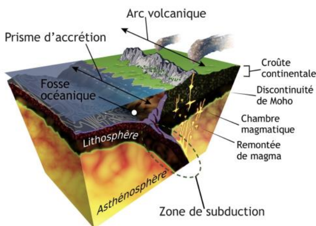
Schéma théorique d'une zone de subduction
